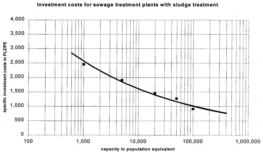
Abb. 3.2: Modellkostenkurve für Kläranlagen
