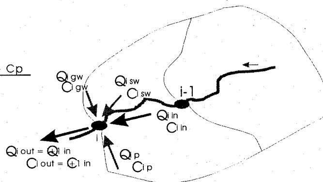
Abb. 2.3: Schematische Darstellung des Box-Konzeptes für den Stofftransport/Stoffrückhalt im Flußsystem (nach WITTGREN & ARHEIMER 1995)
