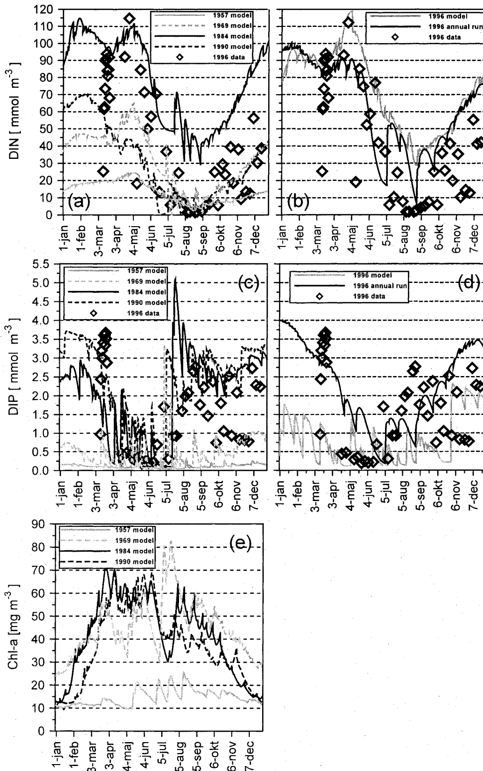
Abb. 4.5: Simulierter Jahreslauf von a) DIN c) DIP, e) Chl a in der Wassersäule des Oderhaffs; ausgewählte Jahre aus einem 47 Jahres-Lauf; b) für N und d) für P geben einen Vergleich zwischen dem Langzeitmodelllauf und einer einjährigen Modellsimulation wieder; die Rauten geben Messungen aus dem Jahre 1996 wieder.
