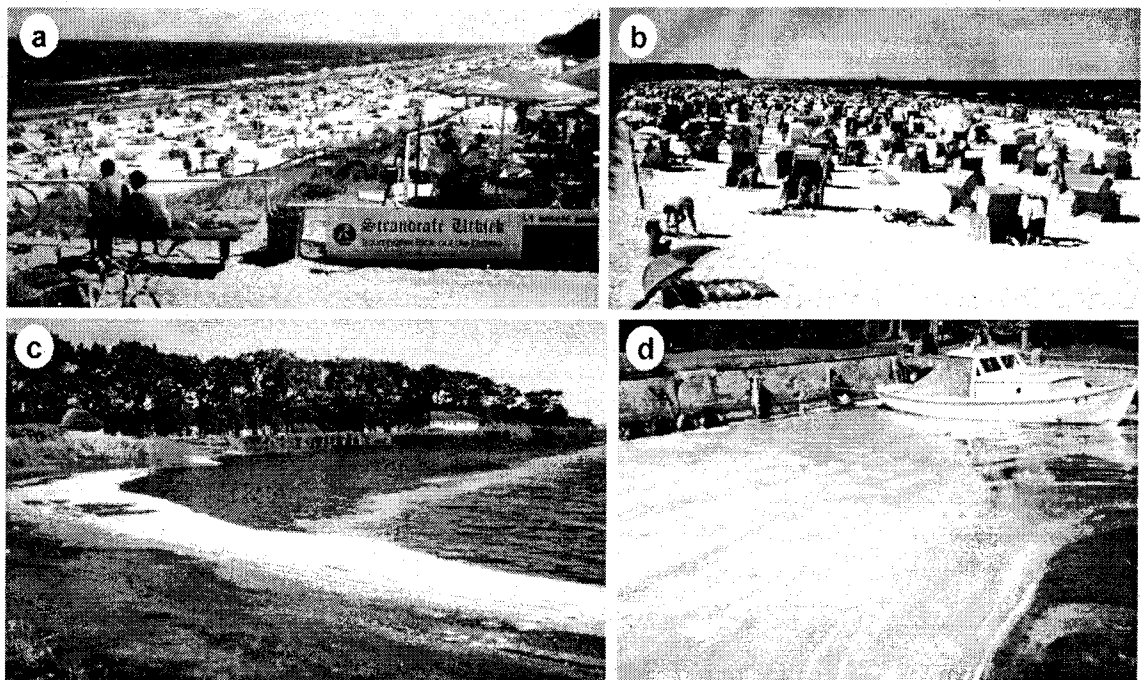
Abb. 1.1 Konflikt Küstennutzung und Wasserqualität: (a,b) Badetourismus in Uckeritz und Ahlbeck (Usedom) im August 1999. Angeschwemmter Algenschaum verursacht durch Massenentwicklung der Blaualgenart (Cyanobakterie) Microcystis (c) im Greifswalder Bodden nahe Lauerbach (Rügen) im September 1999 und (d) nahe Dargen auf der Haffseite von Usedom im August 1999.
