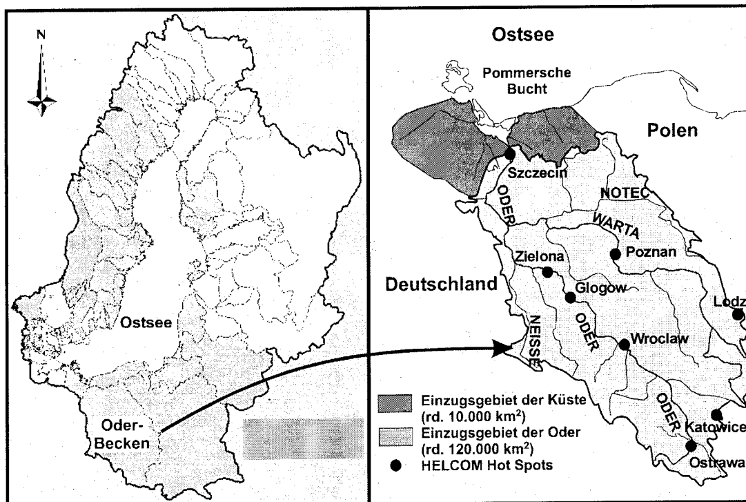
Abb. 1.2 Flußeinzugsgebiete der Ostsee (Quelle: Internet-site of the Institute of Systems Ecology, Stockholm University) und das Odergebiet mit den Belastungsschwerpunkten (Hot Spots) der HELCOM.
