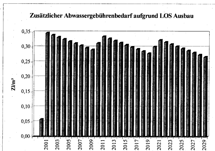
Abb. 3.5: Frachtreduzierung LOS und zusätzlicher Abwassergebührenbedarf
